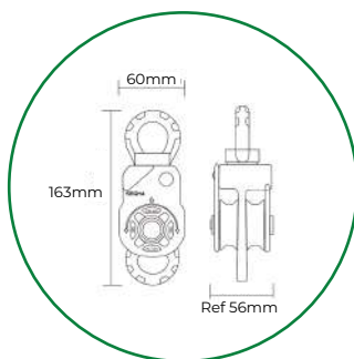
POLEA PEQUEÑA
